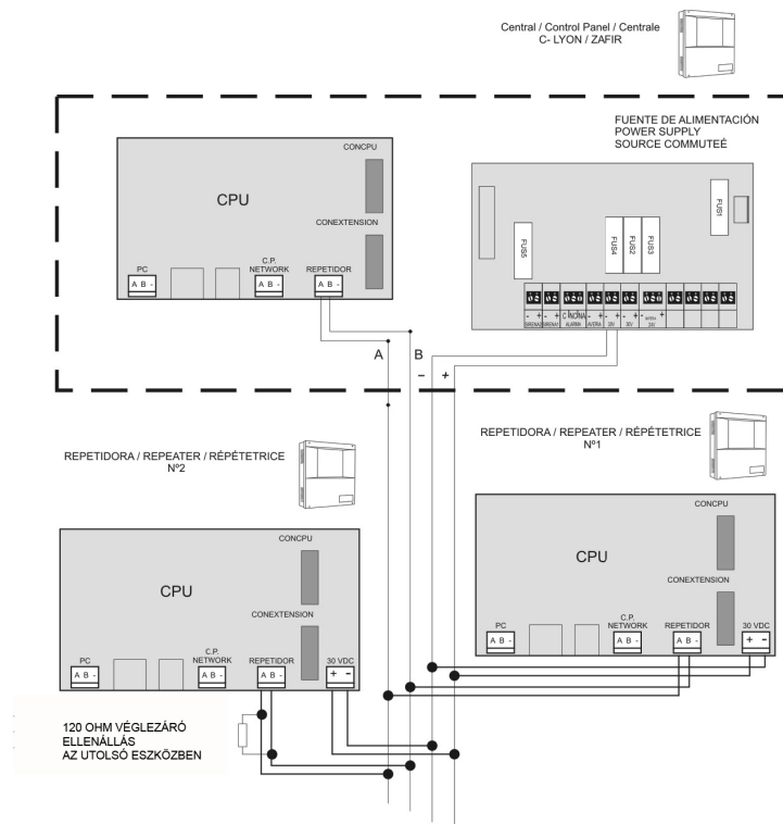
Bekötési rajz (Lyon Control Panel)
