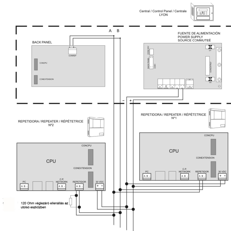
Bekötési rajz (Lyon Control Panel)
